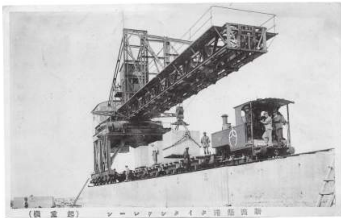
〔絵葉書 新潟築港タイタンクレーン (起重機)〕 新潟築港工事に使用された巨大なクレーン。
